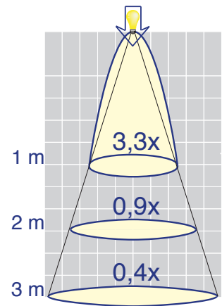
PL115140 (30°) - 3 METER
