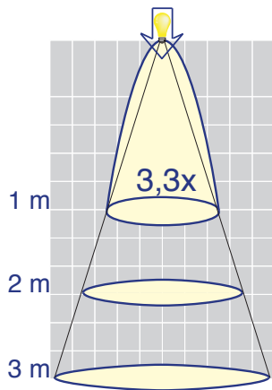
PL115140 (30°) - 1 METER
